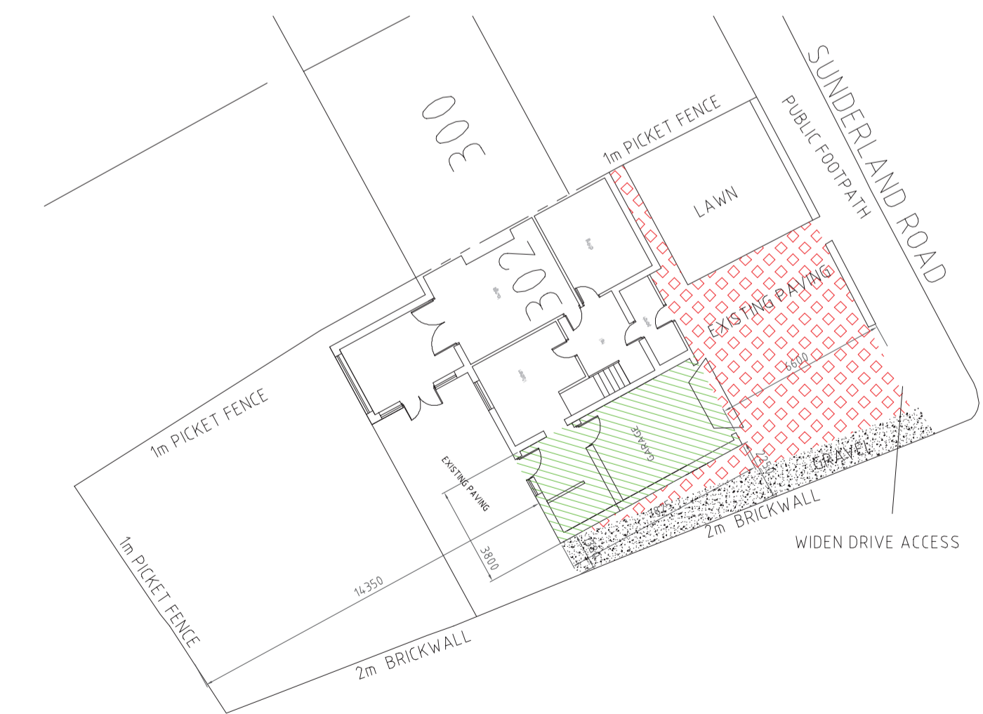
SITE PLAN 1:200
